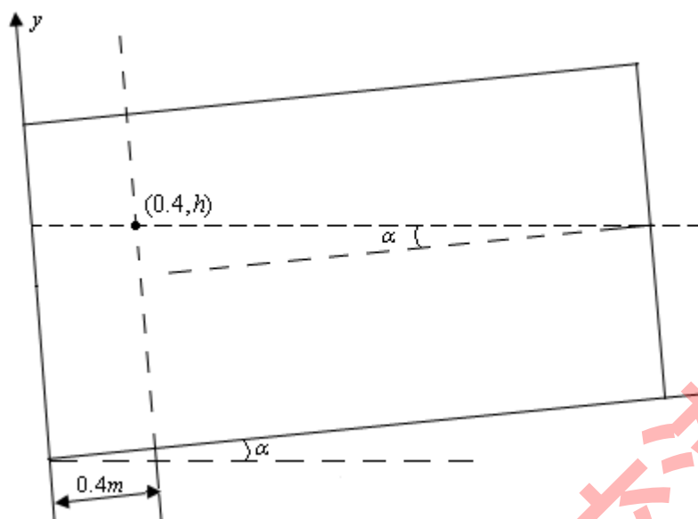
图 2 小油罐纵向截面示意图
