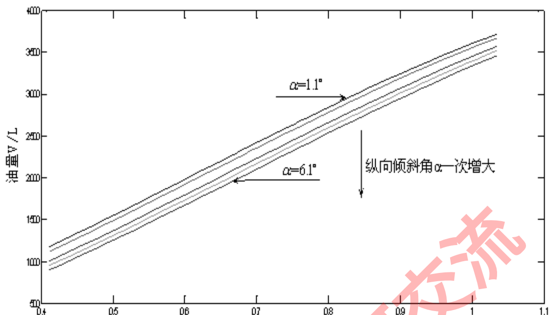
图3 油罐的纵向倾角对其罐容表的影响
