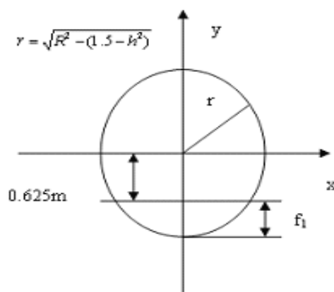
图 8 球罐体横向截面积
